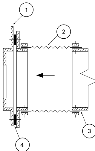
Рисунок 3 - Впуск
