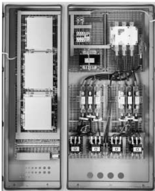
Рис. 2 Панель управления, смонтированная на агрегатах с винтовыми компрессорами, оснащенными модулем UCM-CLD
